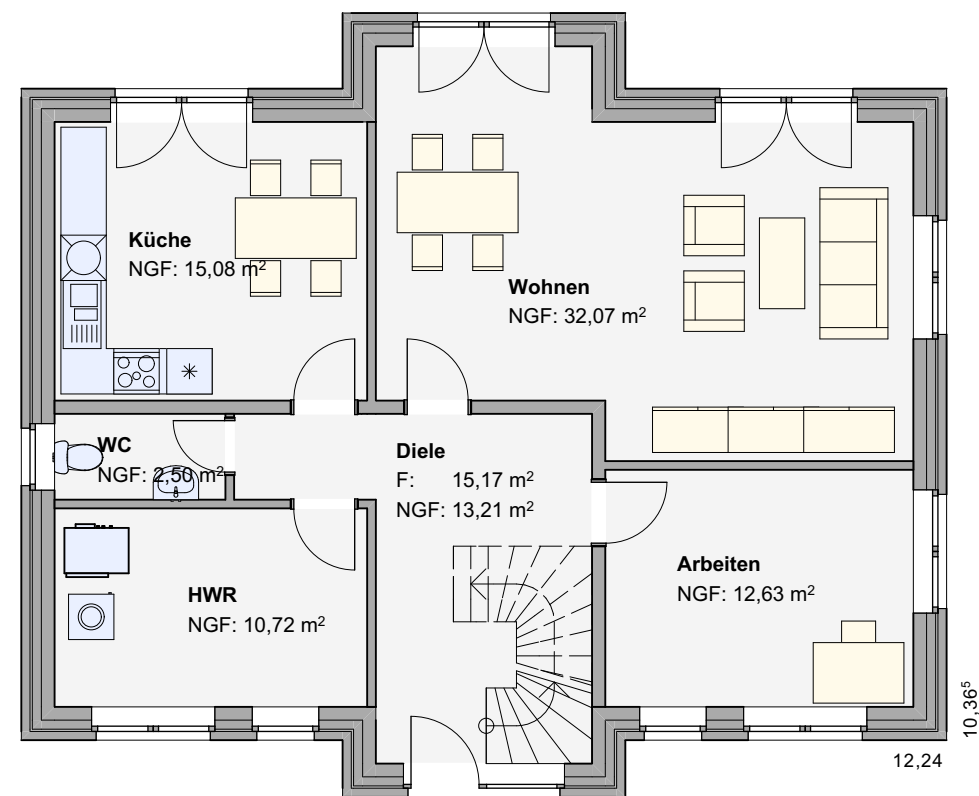
Erdgeschoss
