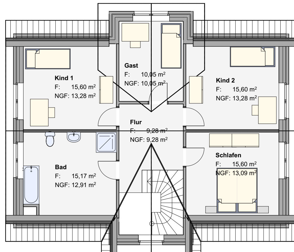
Dachgeschoss
