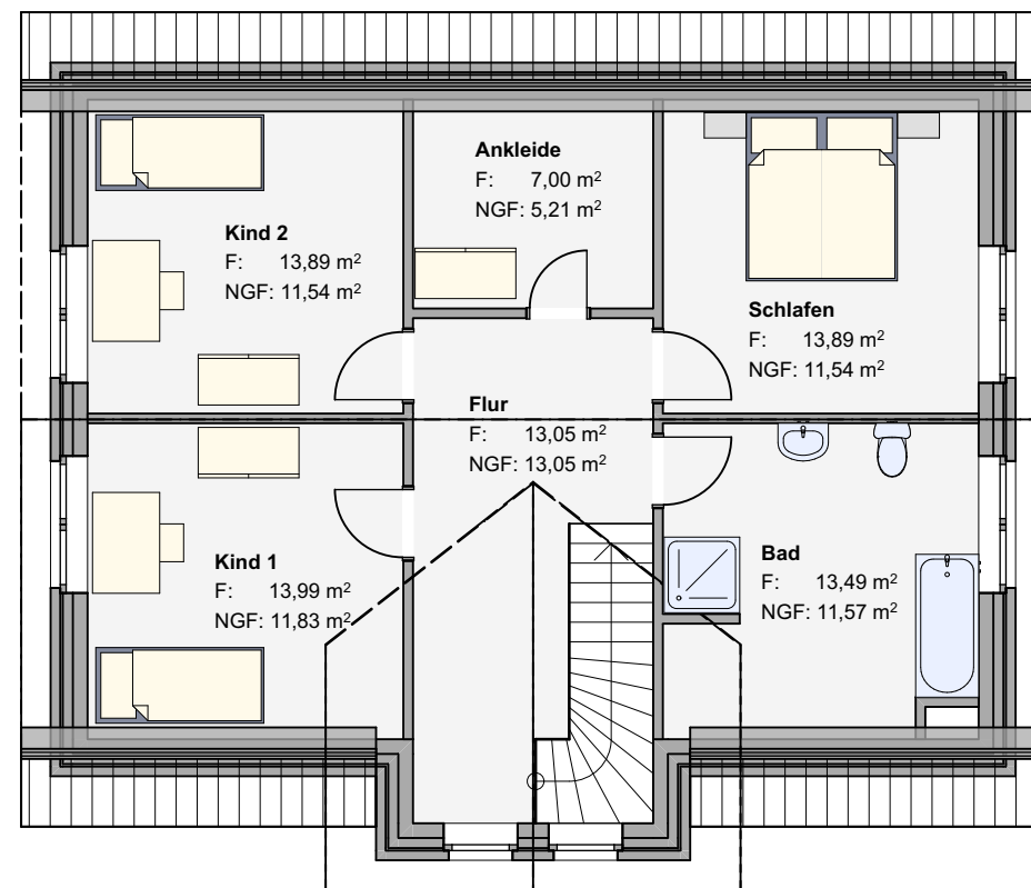
Dachgeschoss
