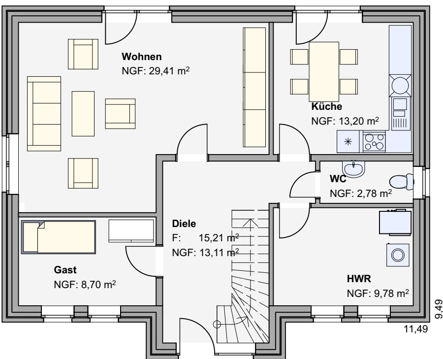
Erdgeschoss
