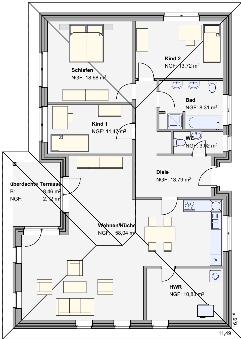
Erdgeschoss
