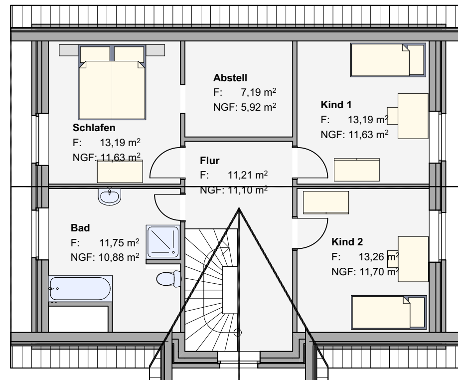
Dachgeschoss
